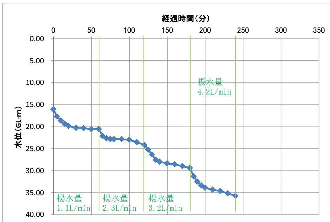
図 4.4.9 段階揚水試験時の水位変化 (No. 17)
